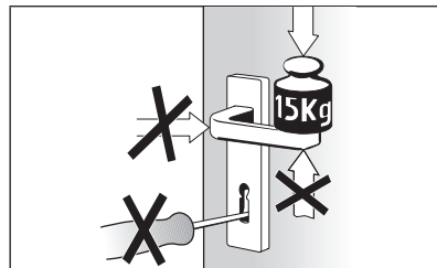
Deurkruk alleen in bedieningsrichting belasten. Max. kracht 150 N. Het slot mag alleen met de bijbehorende sleutel worden gesloten.
